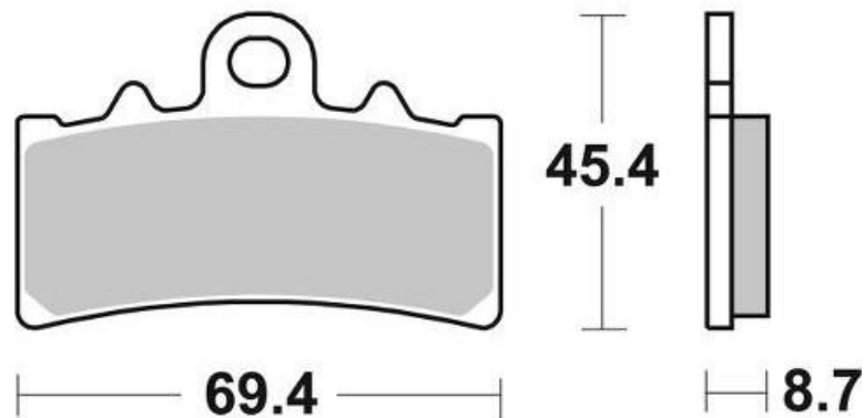
SBS 231MS / WG-8228F8
