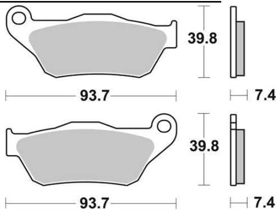
SBS 194MS / WG-7437F8 / WG-8199F8
