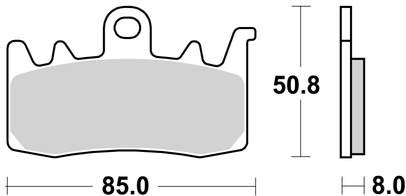
SBS 231MS / WG-8228F8
