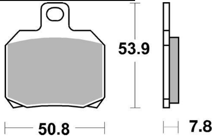
SBS 157MS / WG-7330F8 / WG-8162F8
