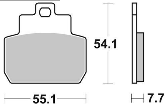
SBS 191MS / WG-7431F8
