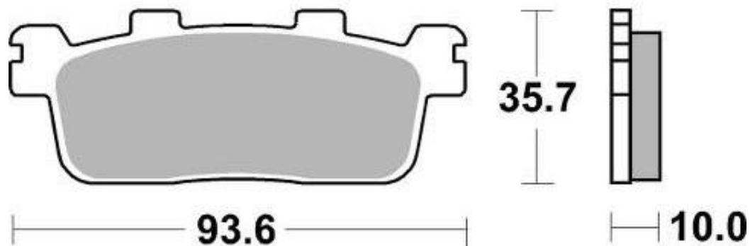
SBS 195MS / WG-7463F8 / WG-8205F8
