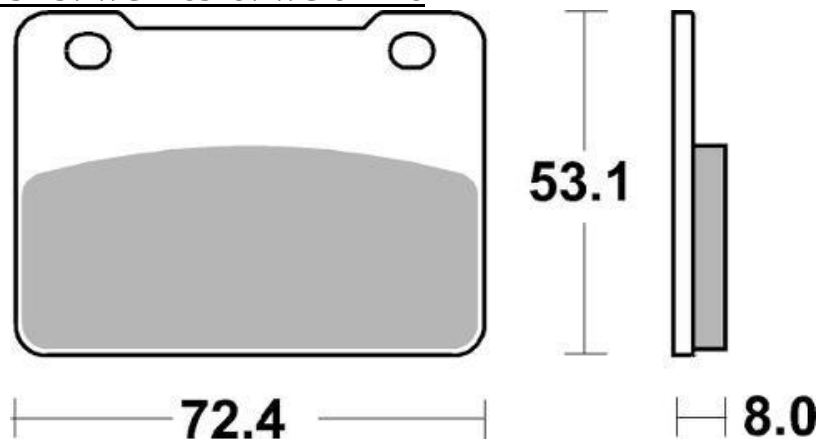
SBS 215MS / WG-7493F8 / WG-8217F8
