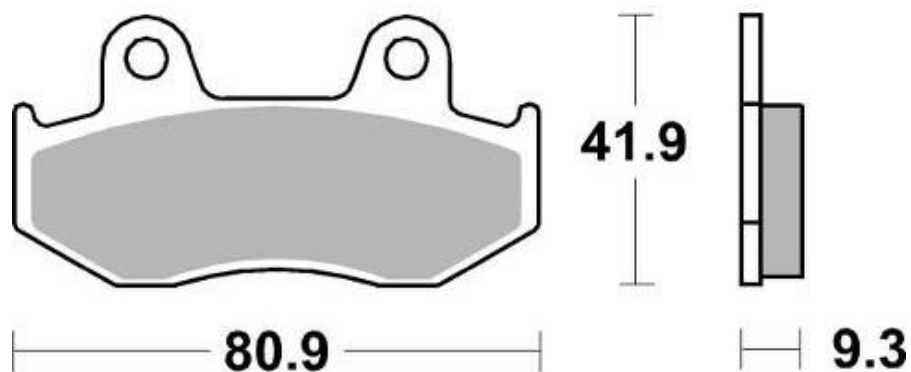
SBS 125MS / WG-7309F8 / WG-8152F8
