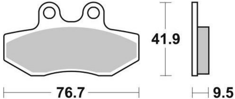
SBS 239MS / WG-7500F8
