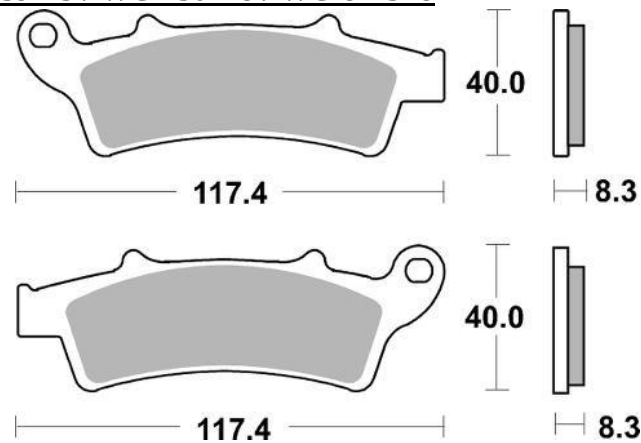
SBS 159MS / WG-7361F8 / WG-8173F8
